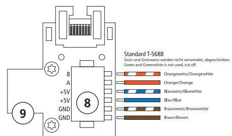
Ansicht H – Verbindungsstandard T-568B.
