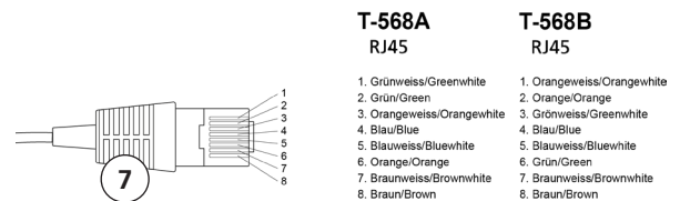
Ansicht F – Unterschiedliche Standards für den Stecker, T-568A und T-568B.
